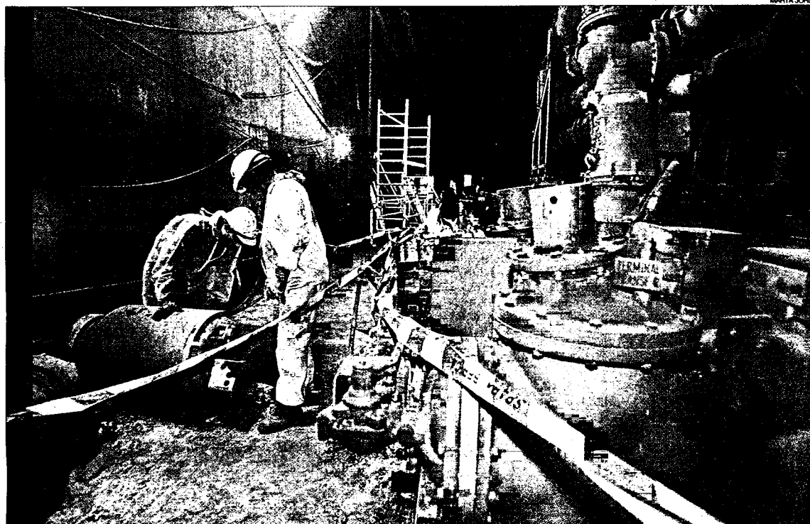
RECONSTRUCCIÓ > Dos operaris treballen a l'interior de la subestació cremada del passeig de Maragall, ahir.
